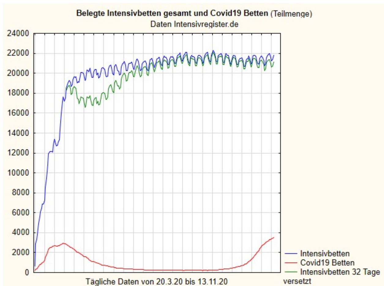
Abbildung 1: Belegung der Intensivbetten in Deutschland (blaue Kurve), Covid-19-Betten als Teilmenge davon (rote Kurve) und Intensivbettenbelegung um 32 Tage (Covid-19 Gipfel) zeitversetzt (grüne Kurve)
